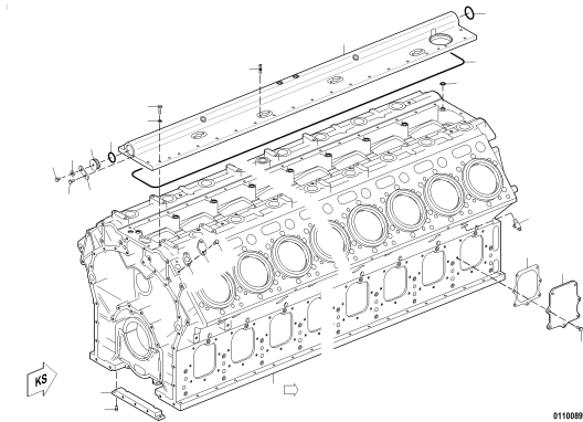
CRANKCASE W/COVER X00019248
